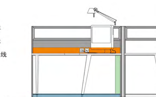
走线示意图
